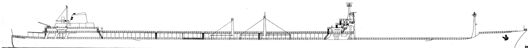
„Idemitsu Maru“ (M 1 : 1.500)
